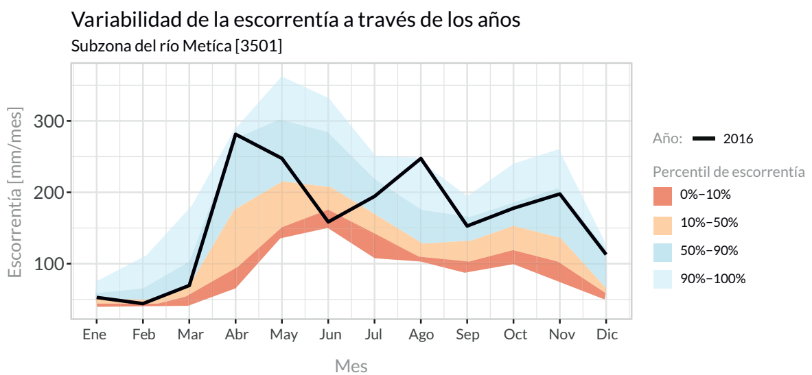
• Figura 29. Variabilidad en la escorrentía en el año 2016 de la subzona 3501, con base en los resultados del modelo DWB.
